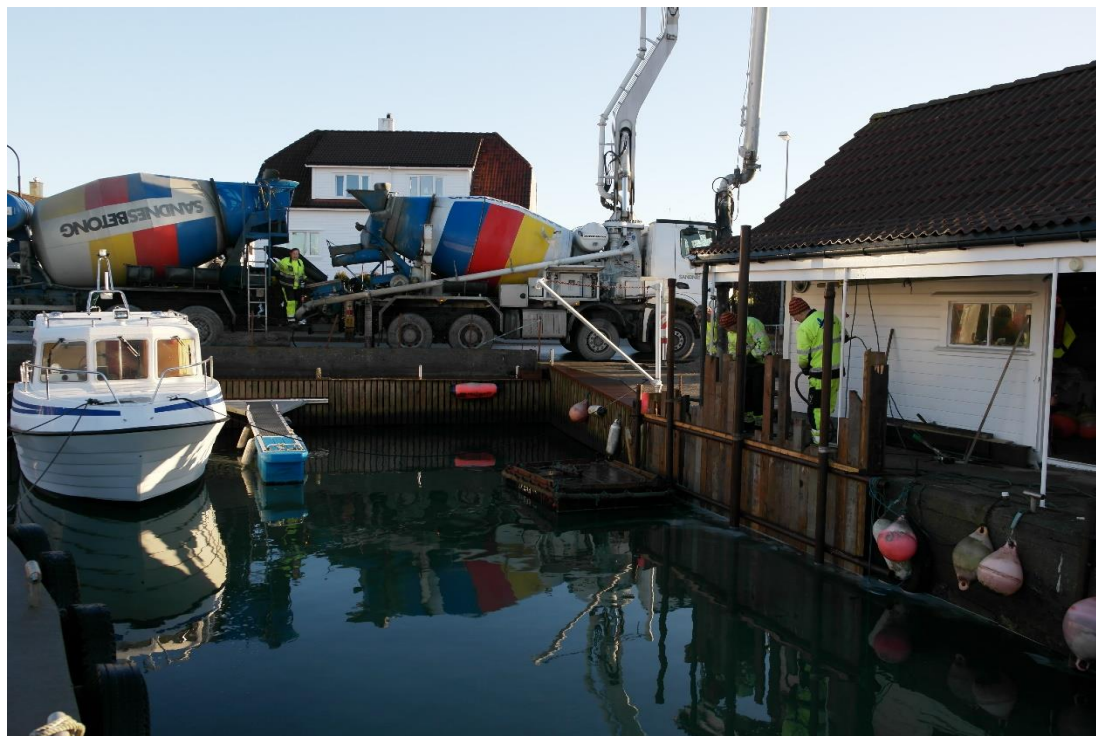
Figur 3 – Støp
