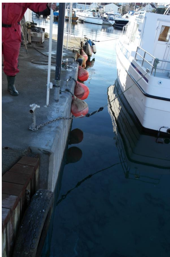
Figur 4 - Ferdig støp
