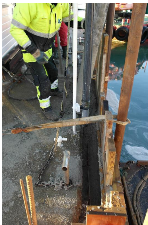
Figur 3 – Støp
